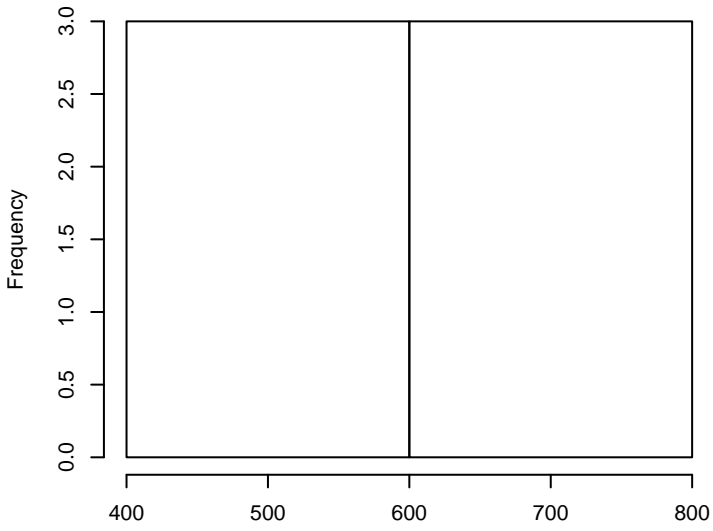
Glu
