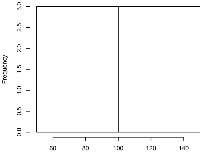
Gln
