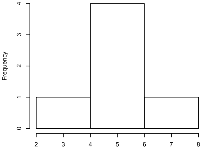
Met
