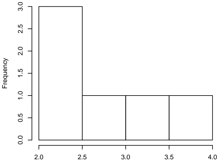
Orn
