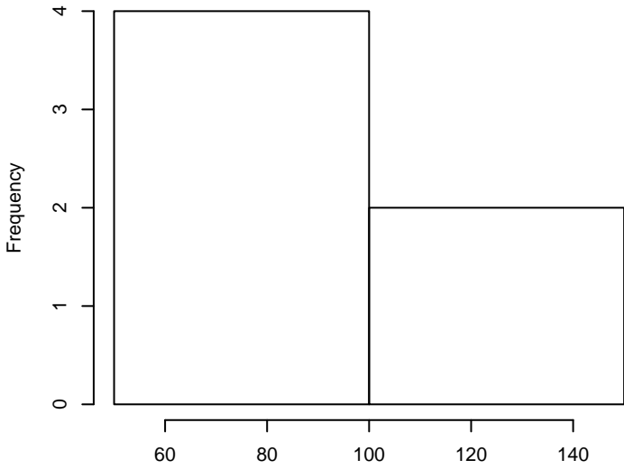
Asp
