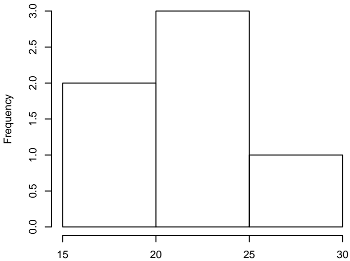
Thr
