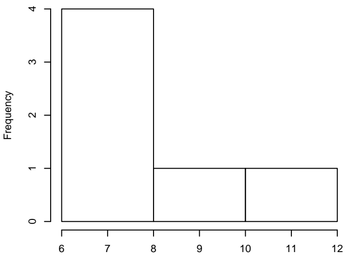
Phe
