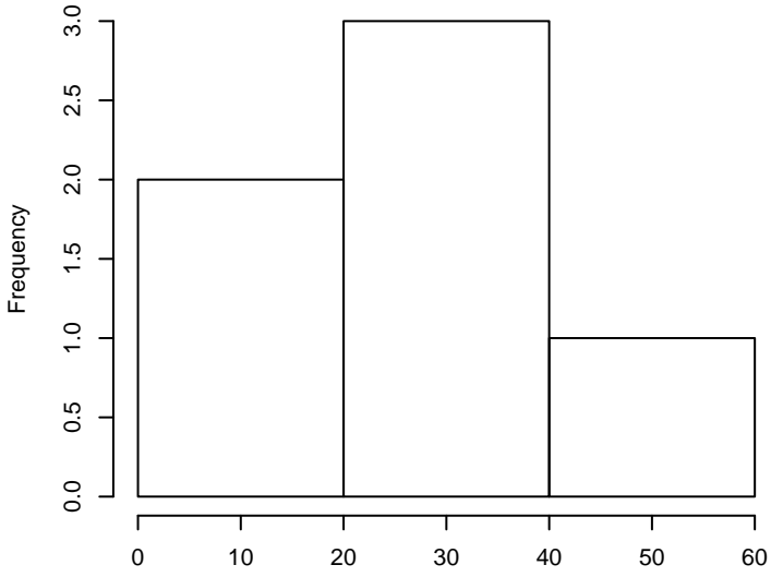
Ser
