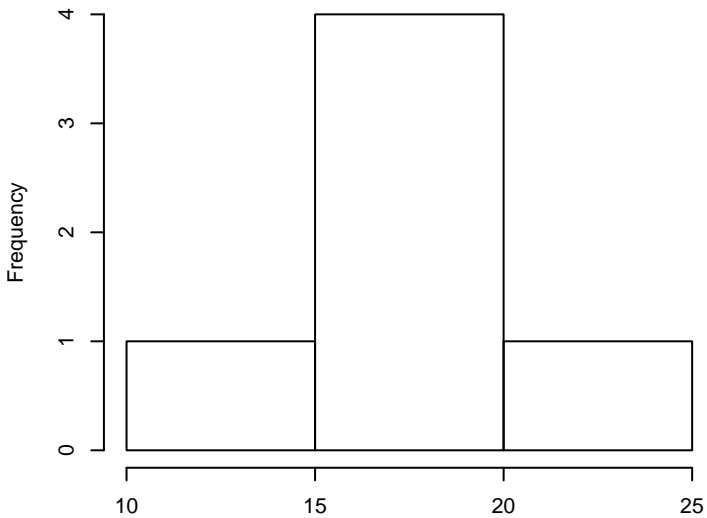
Ile
