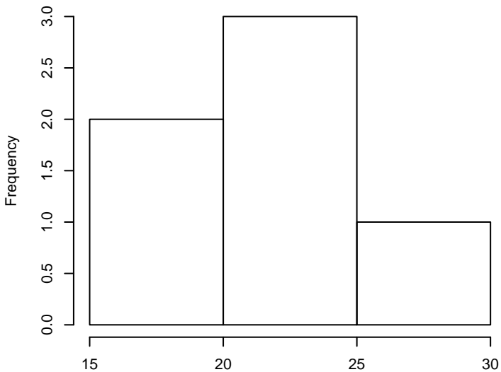
Leu
