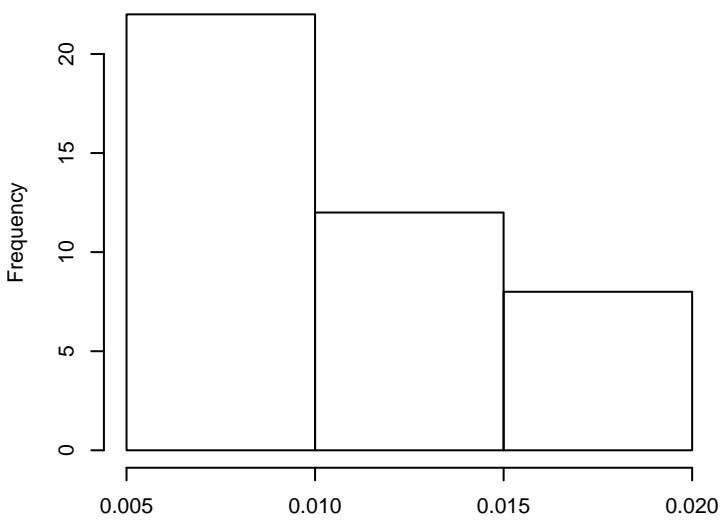
Thr
