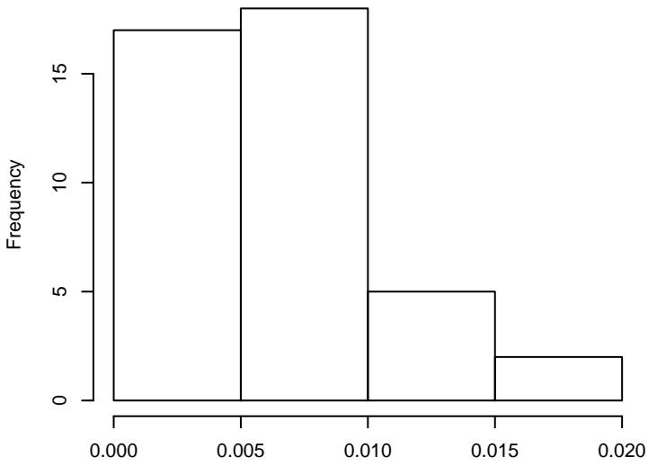
Orn
