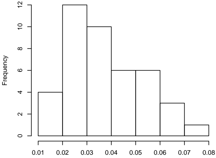
Glu
