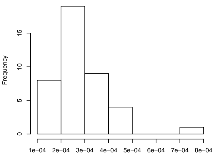
Cit
